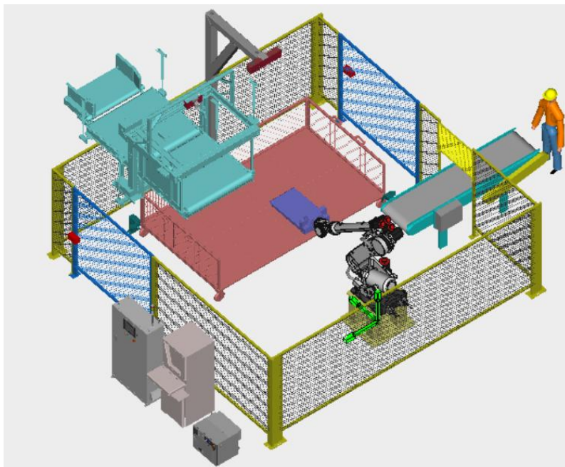
机械手臂智能装载系统布局图
